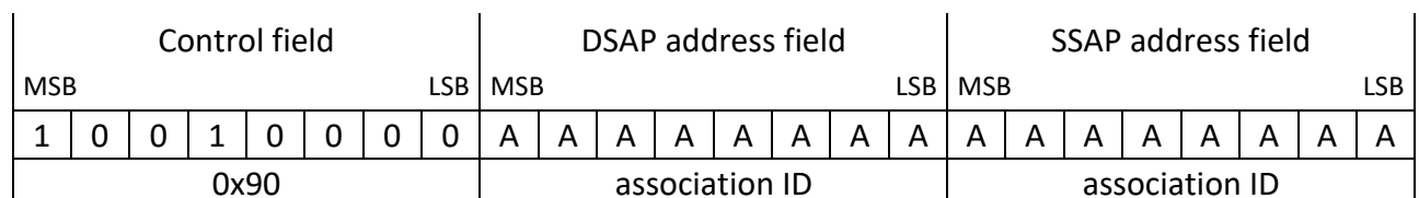
Rysunek 1 Nagłówek protokołu LLC w profilu PRIME PLC
