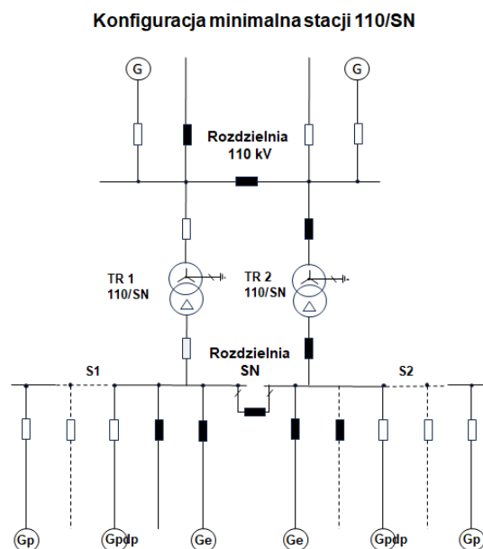
Rys.2. Konfiguracja minimalna GPZ
